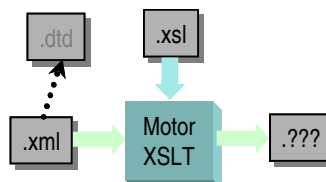
Fig. 5: XSLT.
